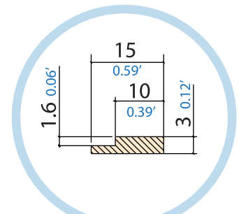
Autoslide SP.4 mm STEEL: MGAUTO0003 BRASS: BFOTTO20X4-N1183
