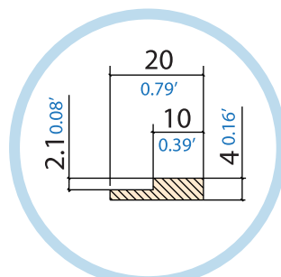
Autoslide SP.3 mm STEEL: MGAUTO0004 BRASS: BFOTTO15X3-N6703
