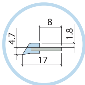
Raschiaolio non protetto COD. BFRASCA6L1MT-000
