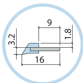
Raschiaolio non protetto COD. BFRASCN1-000000*
