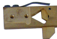
Pattino a scatto in ottone COD. BFSCROOTT60X25X10
