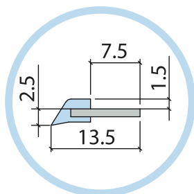
Raschiaolio non protetto COD. BFRASCN3-000000*
